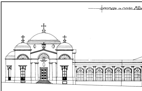
Изо 20. Чертеж проекта церкви: северный фасад 83 , 1912, ЦГАМ.
