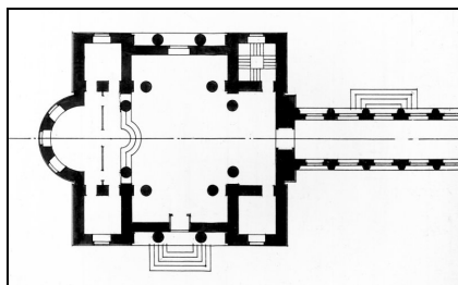
Изо 28. План первого этажа домовой церкви 134 , 1912, ЦГАМ.
