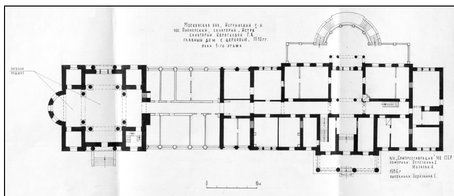
Изо 29. План первого этажа бывшей церкви и усадебного дома 136 , 1986.
