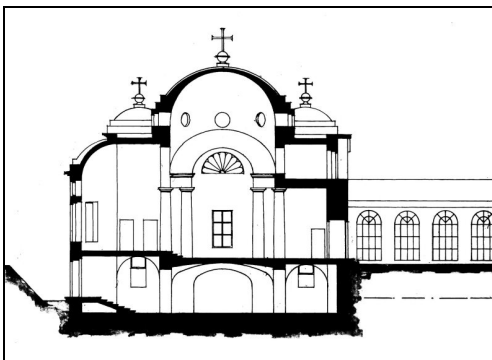
Изо 21. Чертеж проекта церкви: разрез 84 , 1912, ЦГАМ.
