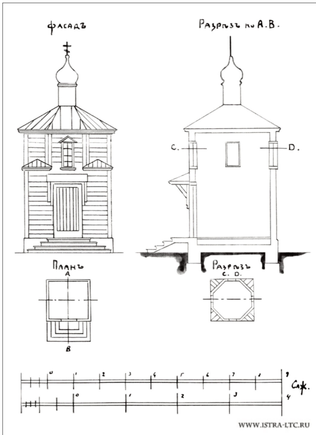
Чертежи новой часовни на Рождественском погосте, 1906 г. [69].
