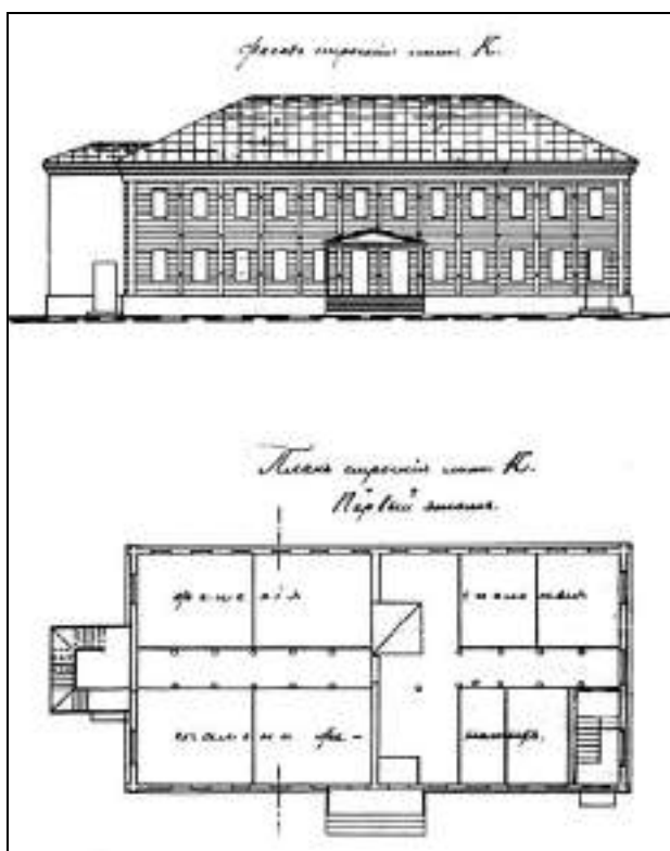
Изо Р-08. Общежитие для рабочих 62 , 1889.
