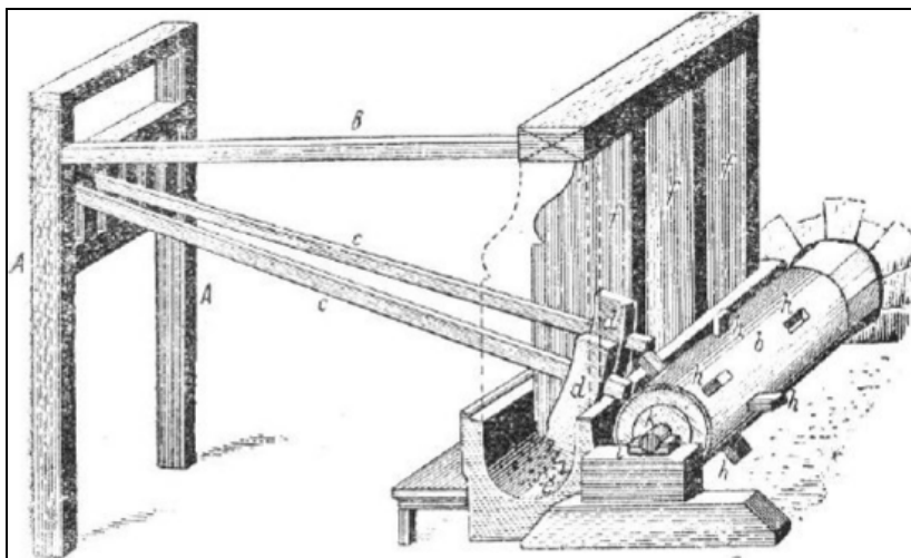
Изо 2–13. Французская сукновальня, 1763.
