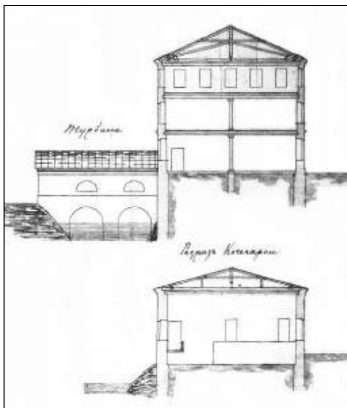
Изо Р–12. Турбина (на канале) и котеларка 66 , 1889.
