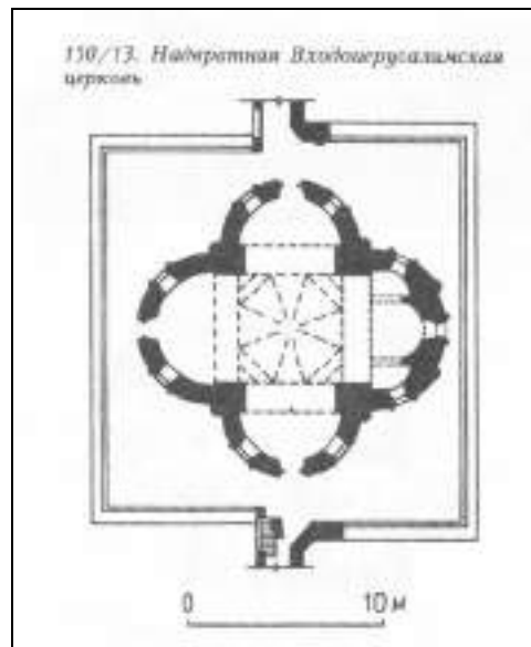
Изо 1–27. План надвратной церкви в Новоиерусалимском монастыре, 1999.
