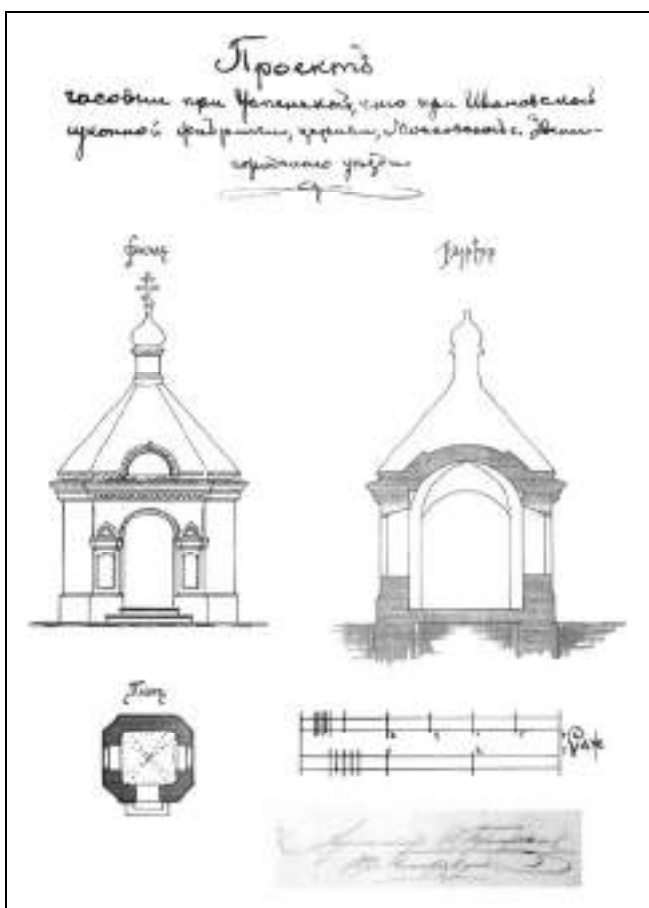
Изо 5-18. Проект второй часовни (утвержден), 1893.
