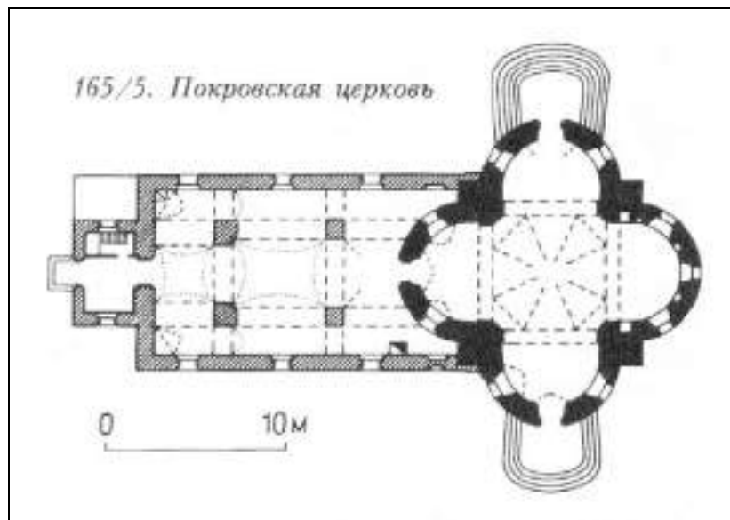
Изо 1–26. План Покровской церкви в Рубцово с выделенным первоначальным объемом 154 , 1999.
